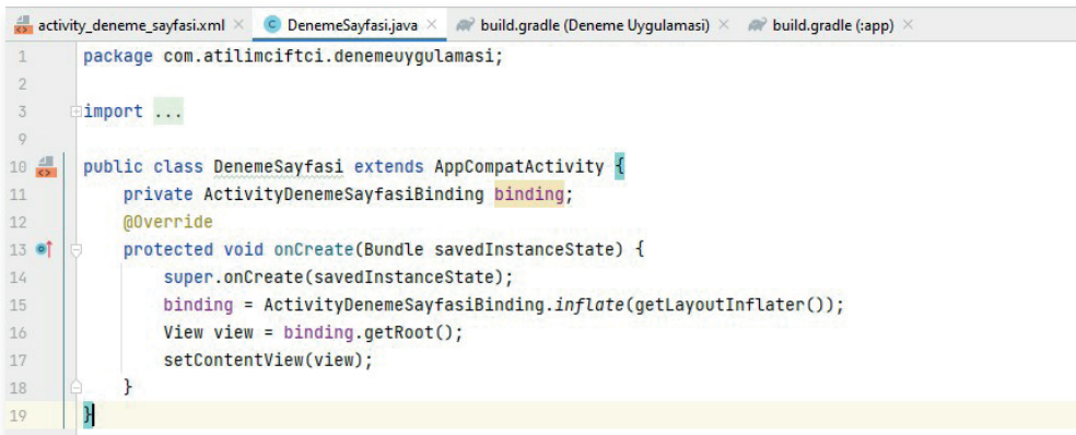
Görsel 6.20: Activity'de viewBinding etkinleştirme
