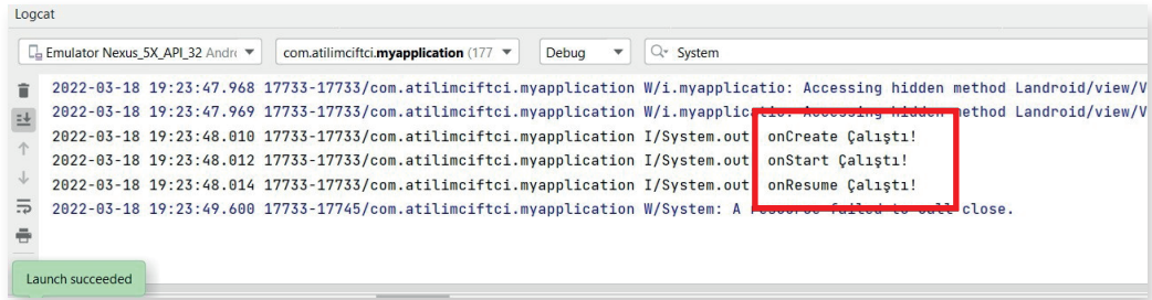
Görsel 6.35: Life Cycle Logcat ekranı
