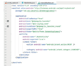
Görsel 6.2: AndroidManifest.xml içeriği
