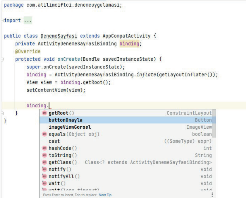
Görsel 6.22: Activity içinde öğelere erişim
