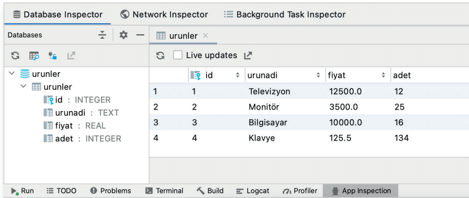
Görsel 7.9: App Inspection eklenmiş kayıtlar
