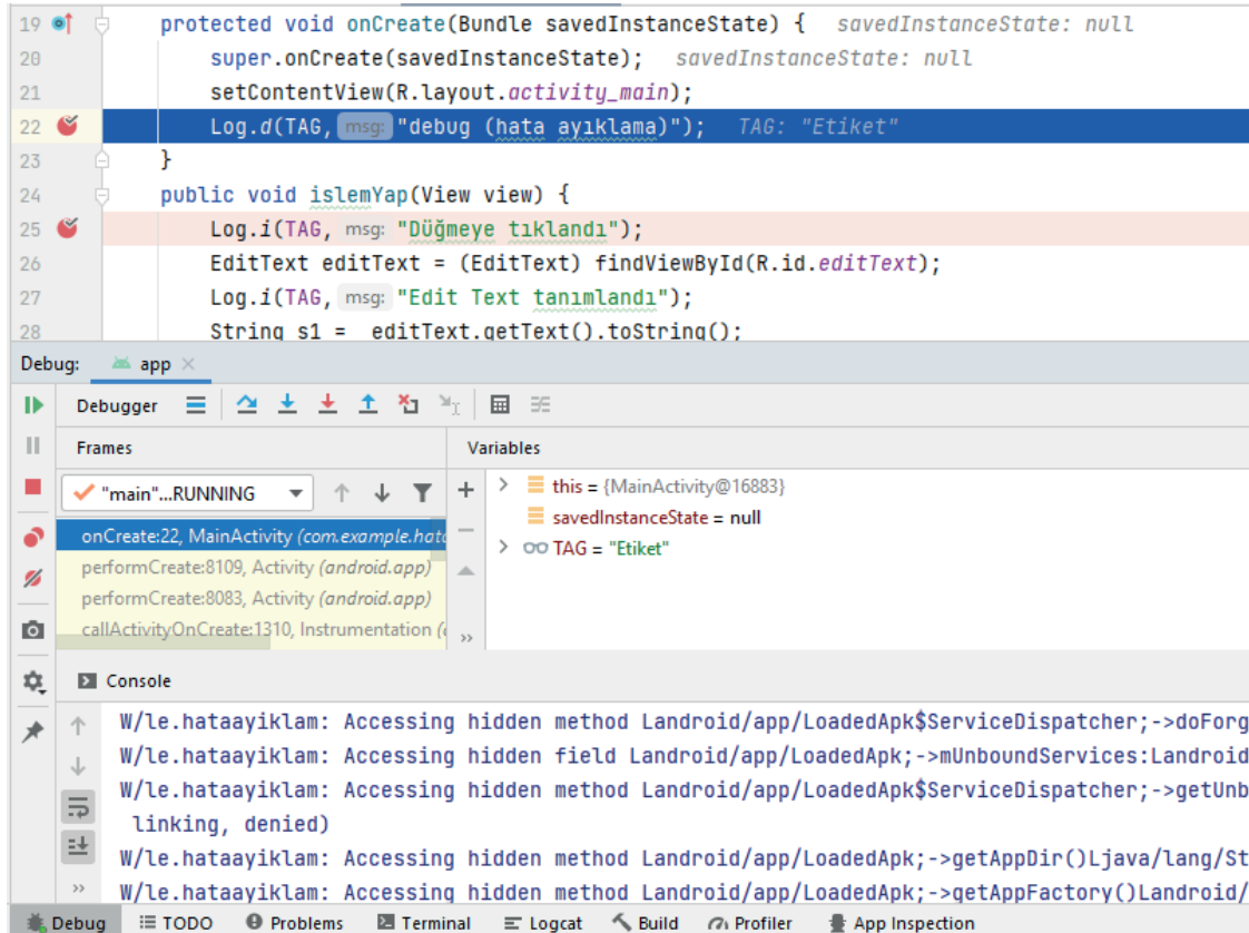
Görsel 3.26. Durak noktası Debug ekranı
