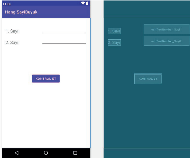
Görsel 4.3: Sayıları karşılaştırma uygulaması tasarımı
