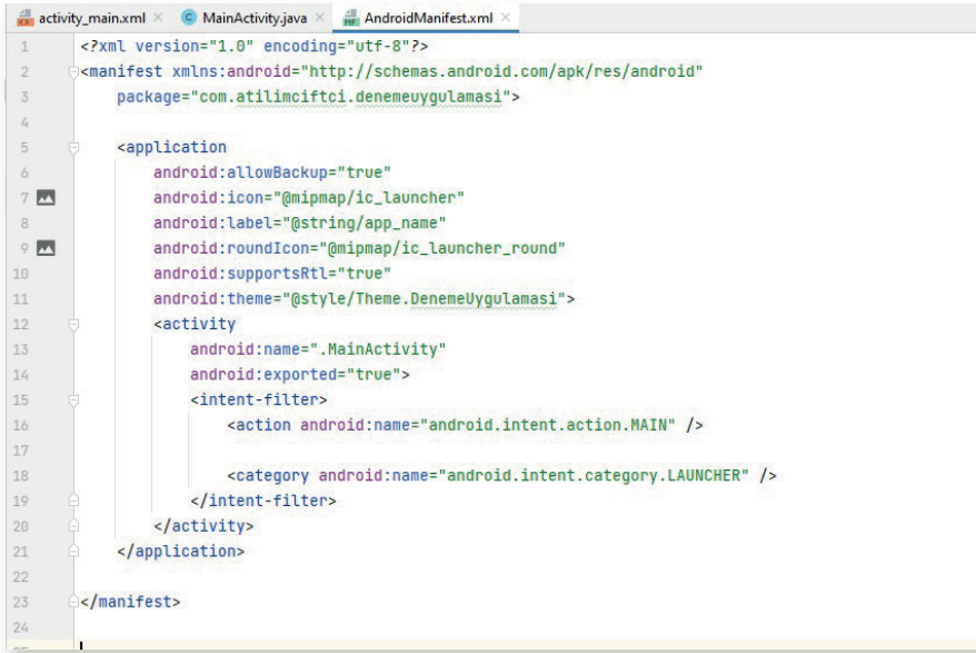
Görsel 6.2: AndroidManifest.xml içeriği
