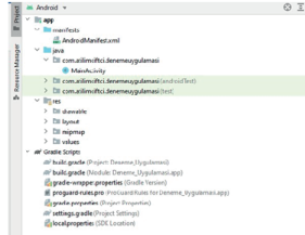
Görsel 6.1: Mobil uygulama geliştirme için Project alanı
