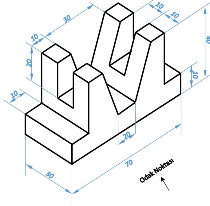
Görsel 1.54: Görünüş çıkarılacak parçanın perspektifi
