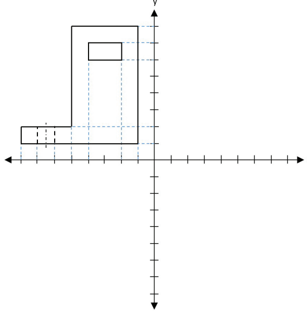
Görsel 1.50: Parçanın ön görünüşünün diedri üzerine yerleştirilmesi
